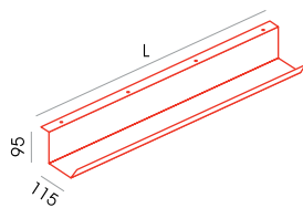
Kabelový koš
